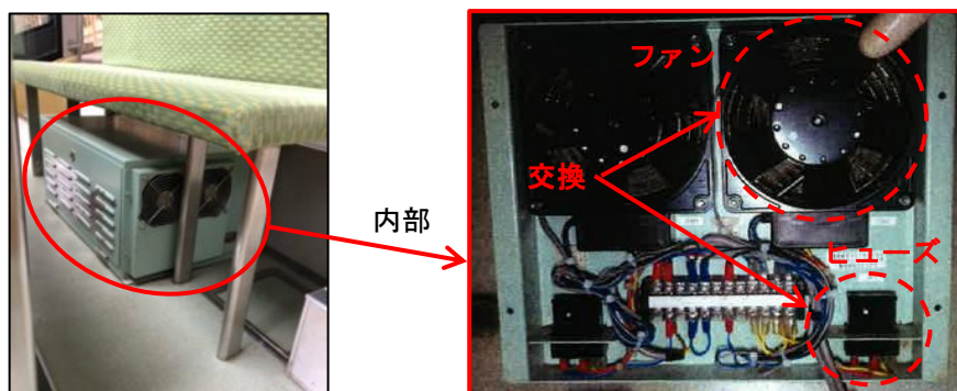
車載用リチウム電源装置
